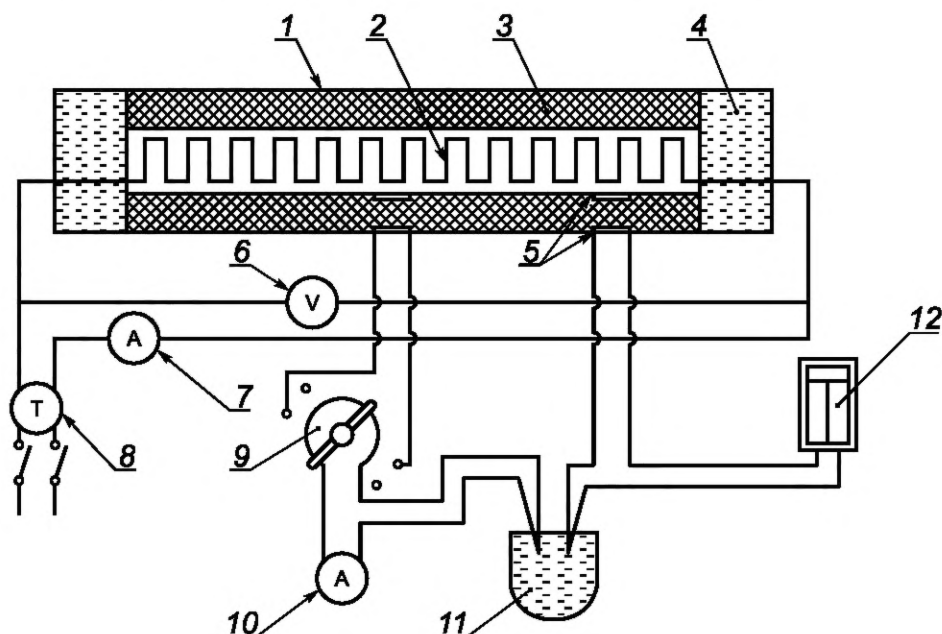
1 — стальная труба; 2 — электронагреватель; 3 — испытываемый материал; 4 — охранная секция; 5 — термодатчики; 6 — вольтметр; 7 — амперметр; 8 — автотрансформатор; 9 — переключатель; 10 — гальванометр; 11 — сосуд со льдом; 12 — самопишущий гальванометр
